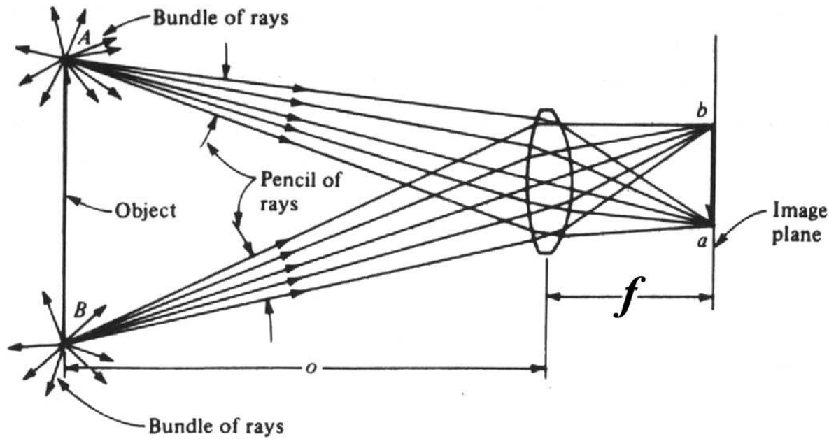
Lente convergente
